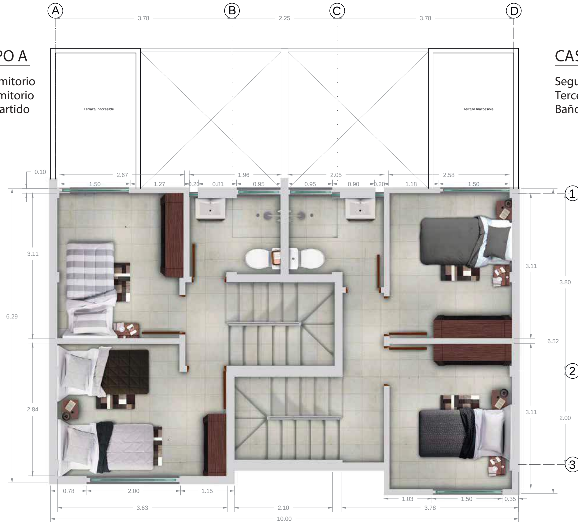
Primera Planta Alta
