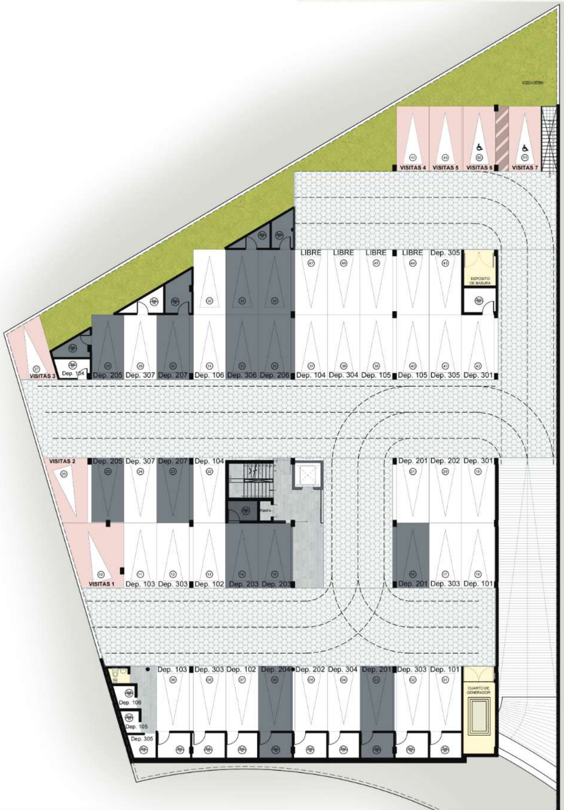
PLANTA SUBSUELO
