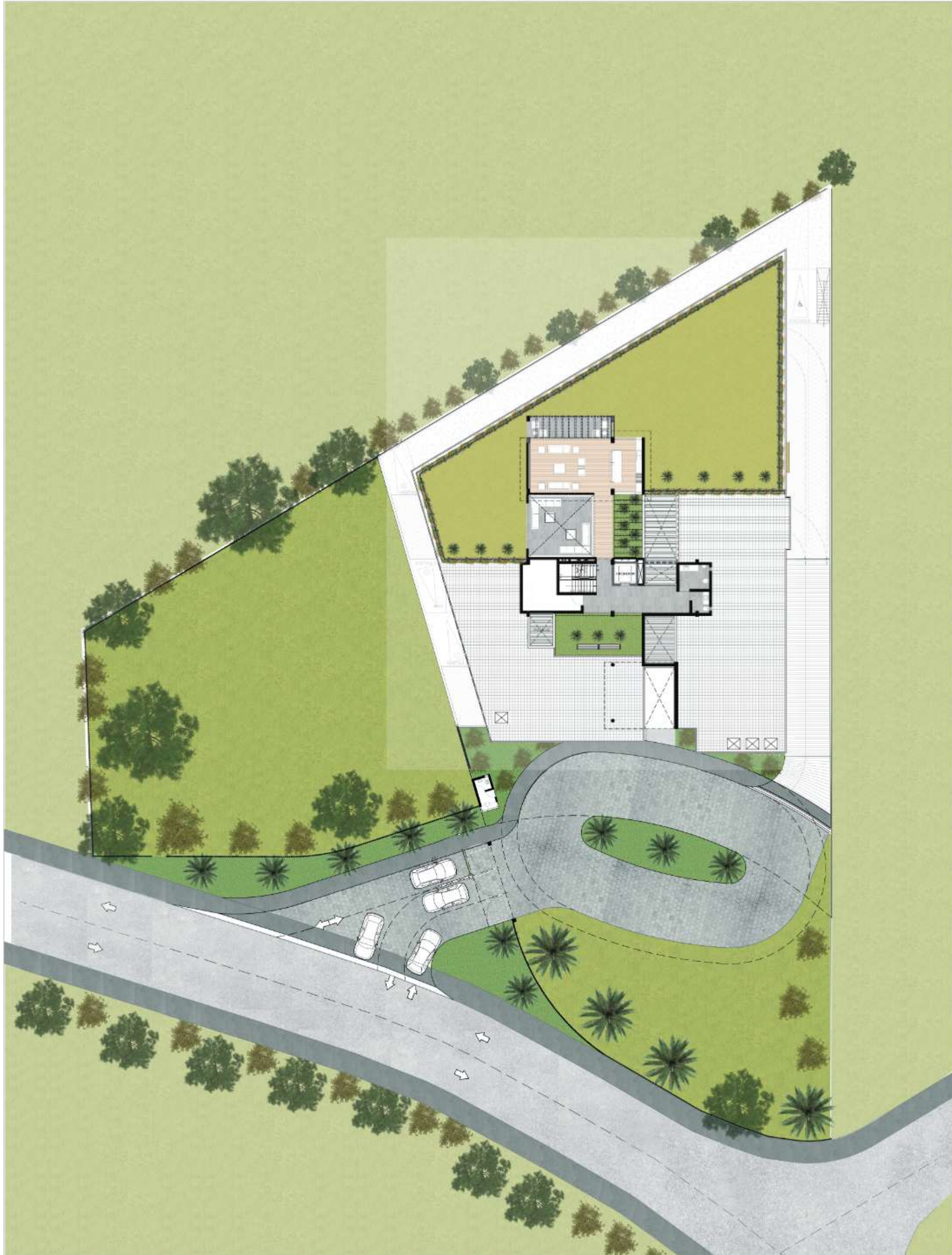
IMPLANTACIÓN - PLANTA CUBIERTA - ROOFTOP
