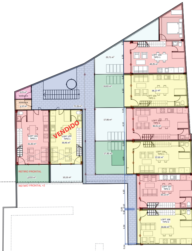
PRIMERA PLANTA ALTA ESCALA: 1:75
